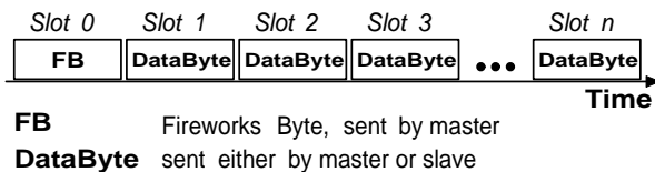
Figure 3: A TTP/A Multipartner Round
