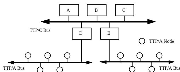
Figure 2: TTP/C and two TTP/A clusters.
